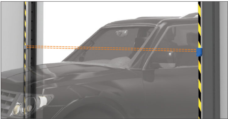
Lichtschanke
